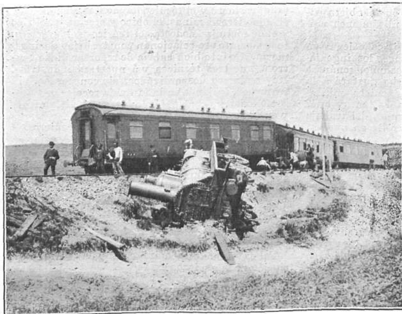
Descarrilamiento del exprés de Sevilla entre Hornachuelos y Palma del Río. Vista tomada por un ingeniero á los dos días de ocurrir el accidente.
