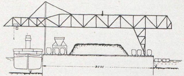
Figura 4.ª—Sección transversal del muelle de combustibles sólidos.
