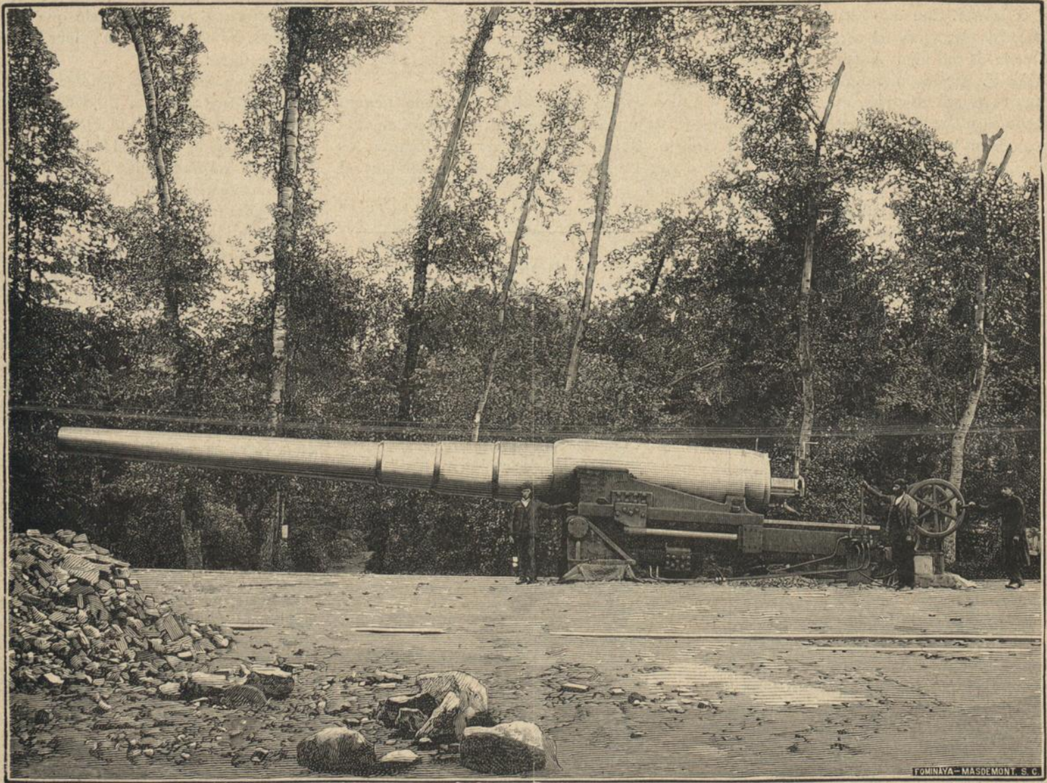
CAÑÓN DE 32 cm. CONSTRUIDO EN TRUBIA PARA EL ACORAZADO PELAYO
