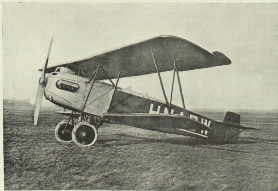
Aeroplano FOKKER C. IV, de reconocimiento
