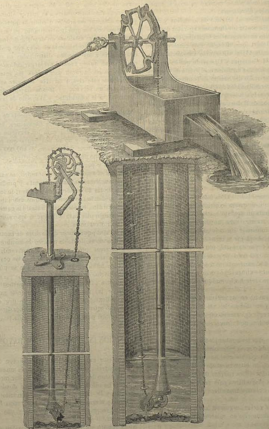
Bomba noria.
