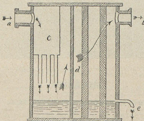
Sección vertical del aparato Baker
