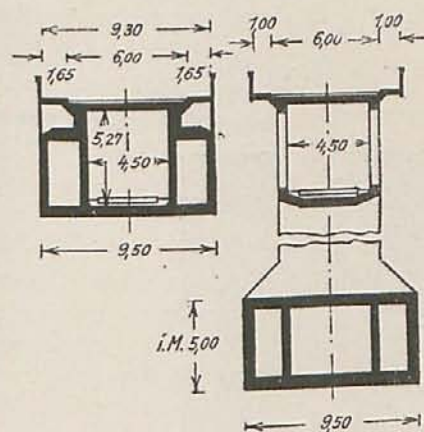
Fig. 16. — Secciones transversales del puente de Plougastel.
