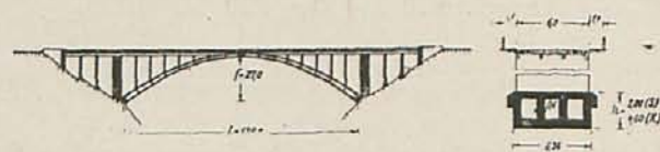
Fig. 10.—Puente sobre el Caille, en Cruseilles.
