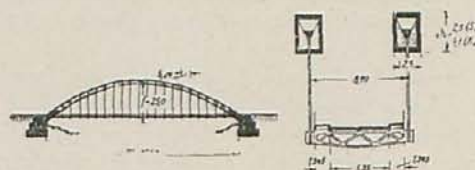
Fig. 9.—Puente sobre el Sena, en St. Pierre du Vauvray.
