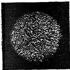
Acero alterado por exceso de calor al templearlo
