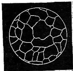
Alambre de acero templado en aceite
