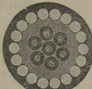
Cable submarino múltiple.
