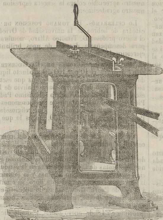
Máquina para hacer ranuras y molduras rectas y curvas.
