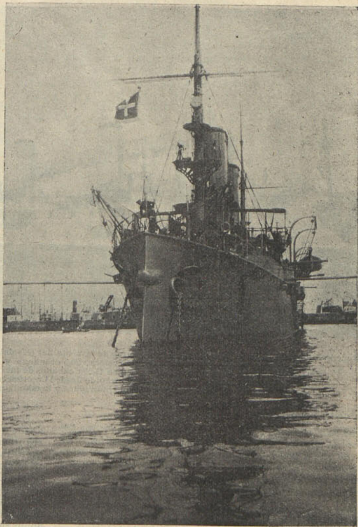
Cruceiro italiano «Umbria» que ancló en este puerto con motivo de la visita del Jefe del Estado. Se botó en 1899. Su casco es de acero y mide 112 metros de eslora, 14 de manga y 7,30 de puntal. Desplaza 7,500 toneladas. Sus máquinas desarrollan 13,500 caballos de fuerza. Su velocidad es de 20 millas por hora. Monta un cañón de 25,4 centímetros, dos de 20,3, 14 de 15,2; 10 de 7,6; seis de 4,7; y dos ametralladoras. Está dotado de 4 tubos lanza-torpedos. Lo tripulan 524 hombres y lo manda un capitán de navío.
