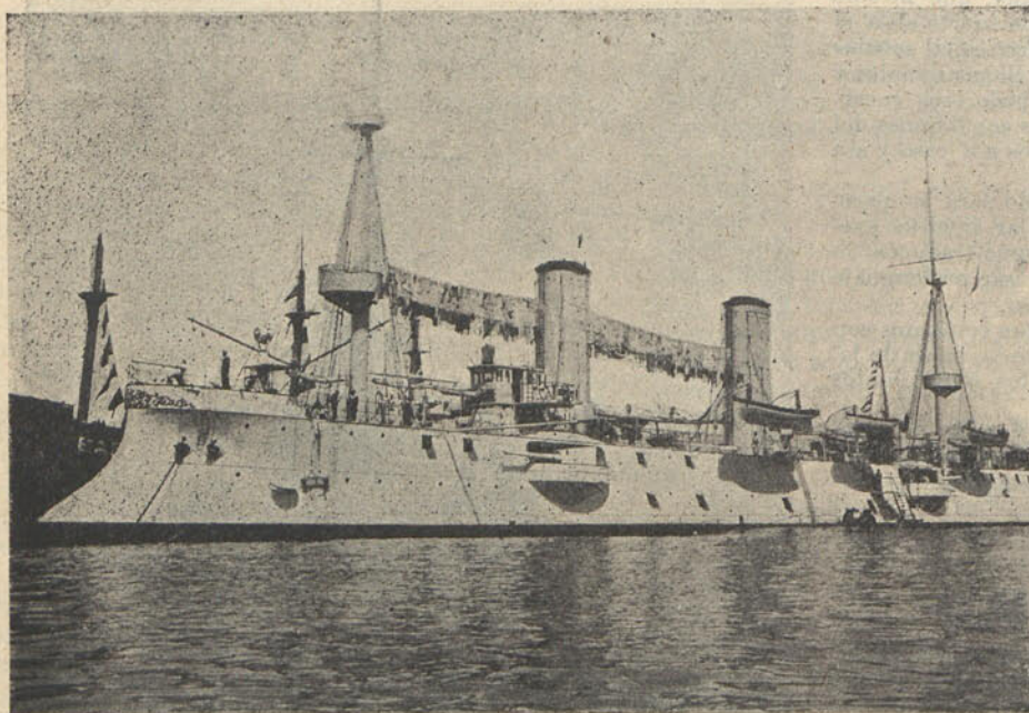
Crucero «Linois», que ancló en este puerto con motivo de la visita del Jefe del Estado. Se botó en 1894. Su casco es de acero. Mide 118 metros de eslora, 20,5 de manga y 8'40 de puntal. Desplaza 11,275 toneladas y sus máquinas desarrollan 14,500 caballos de fuerza. Su velocidad es de 18 millas por hora. Monta 14 cañones de tiro rápido desde 14 centímetros á 37 milímetros. Tiene 4 tubos lanza-torpedos. Lo tripulan 240 individuos y lo manda un capitán de fragata.
