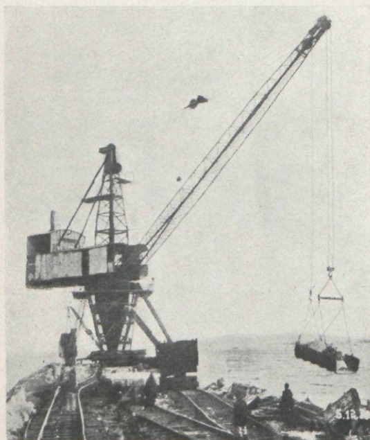
Figura 3.ª—Grúa Pillar, especialmente proyectada para la construcción del rompeolas principal del puerto de Haifa.
