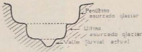
FIGURA 9.—ESQUEMA DE UN VALLE EN U
