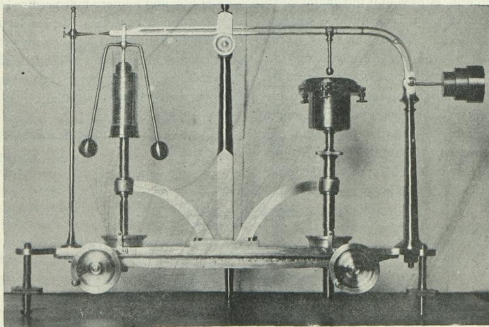
Dinamómetro de balanza para ensayos físicos del tabaco (a un \frac{1}{4} de su tamaño).
