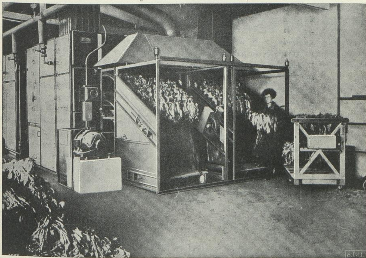
Máquina de doble carga. Como se deposita el tabaco salido del secadero con la suficiente humedad para ser manejable. Parte anterior de la máquina.
