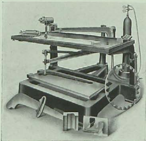
Maquina Perfiladora Num. 61 con movimiento automatico
