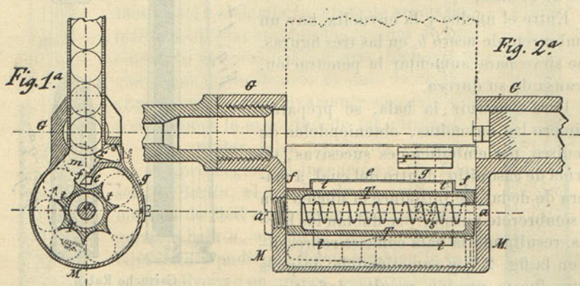
Repetición Mannlicher.
