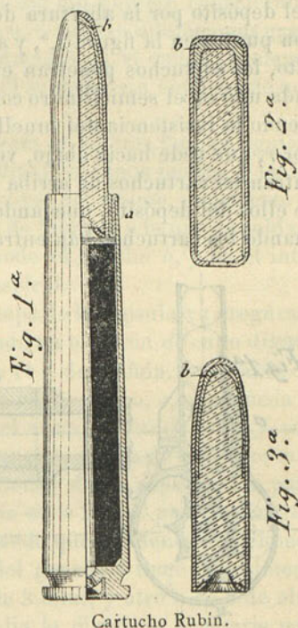
Cartucho Rubin.
