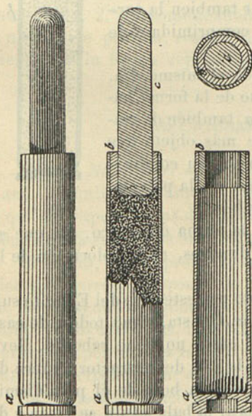
Cartucho Schulhof.
