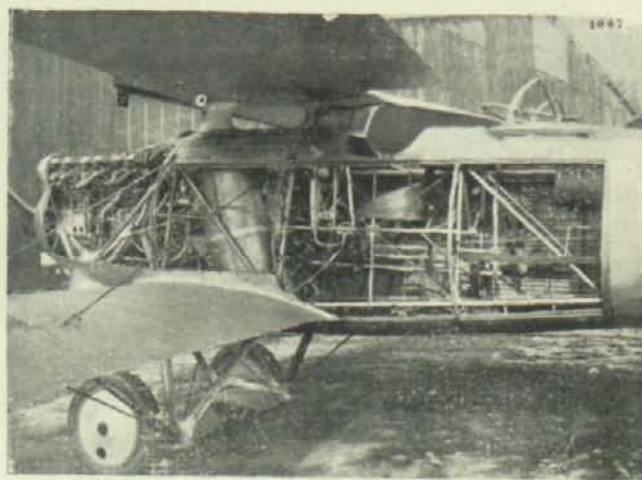
Disposición interior del avión.
