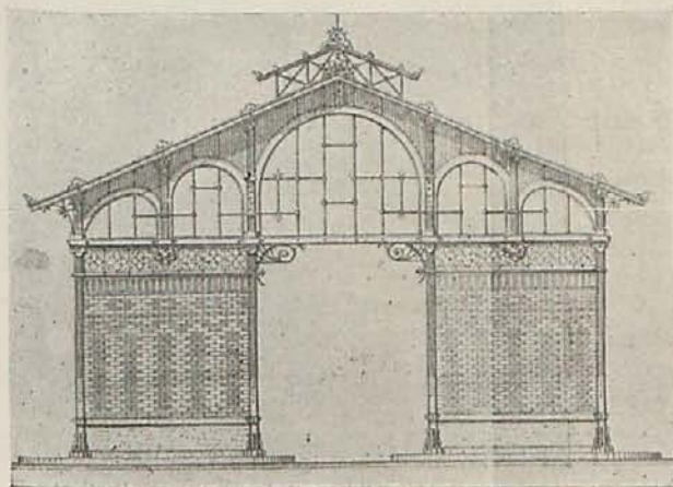
Proyecto de los tinglados para el muelle de Palma.
