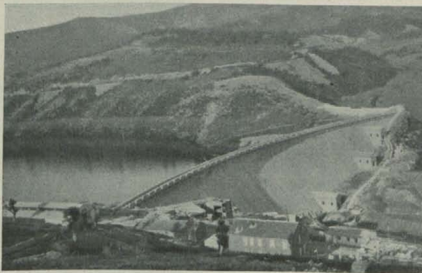
Pantano del Arlanzón.—Vista general de la presa por el paramento de aguas abajo. Julio 1933
