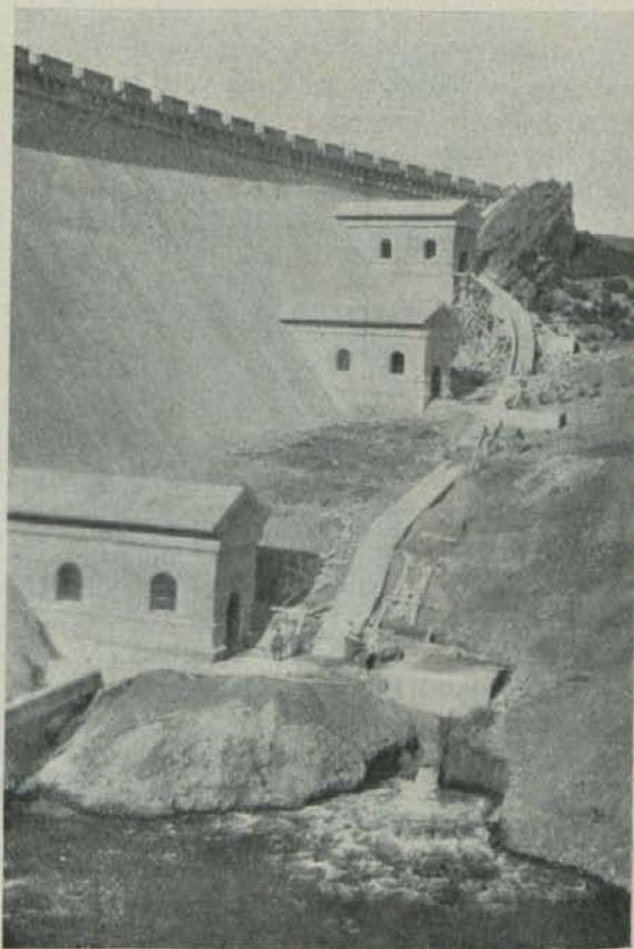
Pantano del Arlanzón.—Casetas de toma de agua y tubería de unión de tomas
