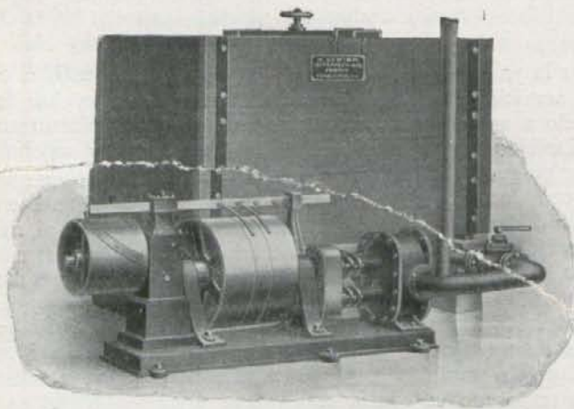
Fig. 5. — Aparato de tñir para trapos
