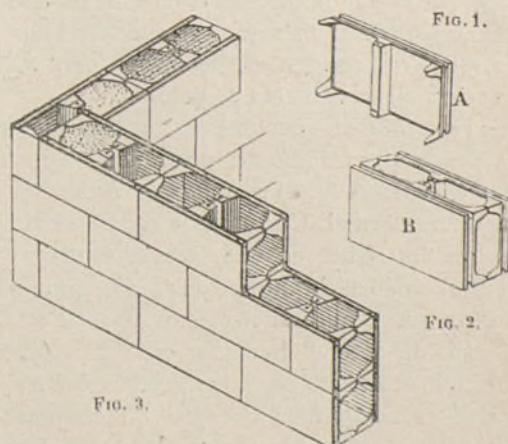
Fig. 1 a 3.—Elementos «doble C» y detalle de un muro construido con elementos de este género.
