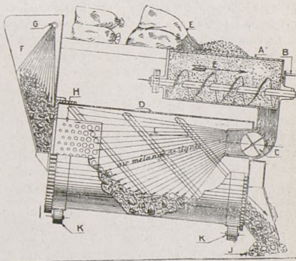
Fig. Corte longitudinal del aereo-amasador por el cilindro mezclador y el dispositivo de llegada de los aglutinantes. A, tamiz.—B, manivela de dosificación.—C, ventilador.—D, tambor mezclador.—E, aglutinantes.—F, tolva para arena y grava.—G, agua.—H, tambor separador.—J, mezcla terminada.—K, poleines de rodadura.—L, angulares de mezcla.
