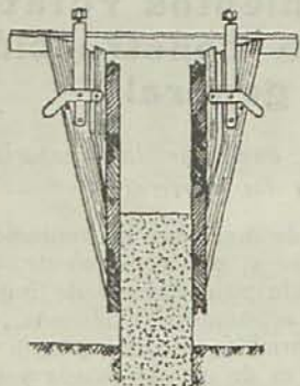
Encofrado para hormigón colado o apisonado
