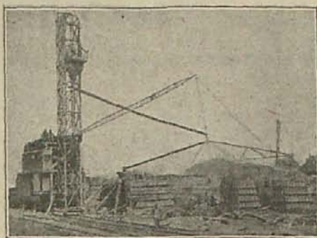
Fig. 1. — Instalación móvil estacionada para verter hormigón. La torre aparece calzada con maderos
