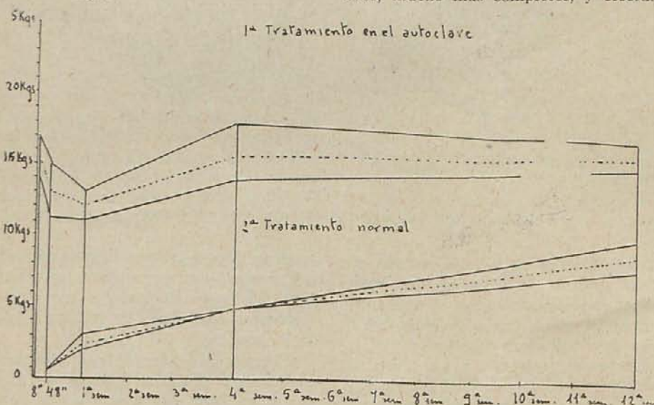
Fig. 1. Resistencia a la ruptura por tracción de las probetas de mortero de cal hidráulica
