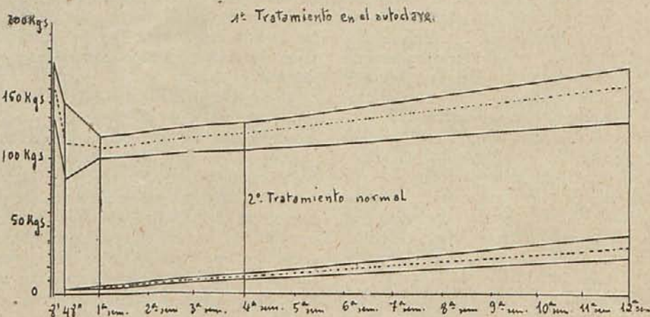
Fig. 2. Resistencia a la compresión de las probetas de cal hidráulica
