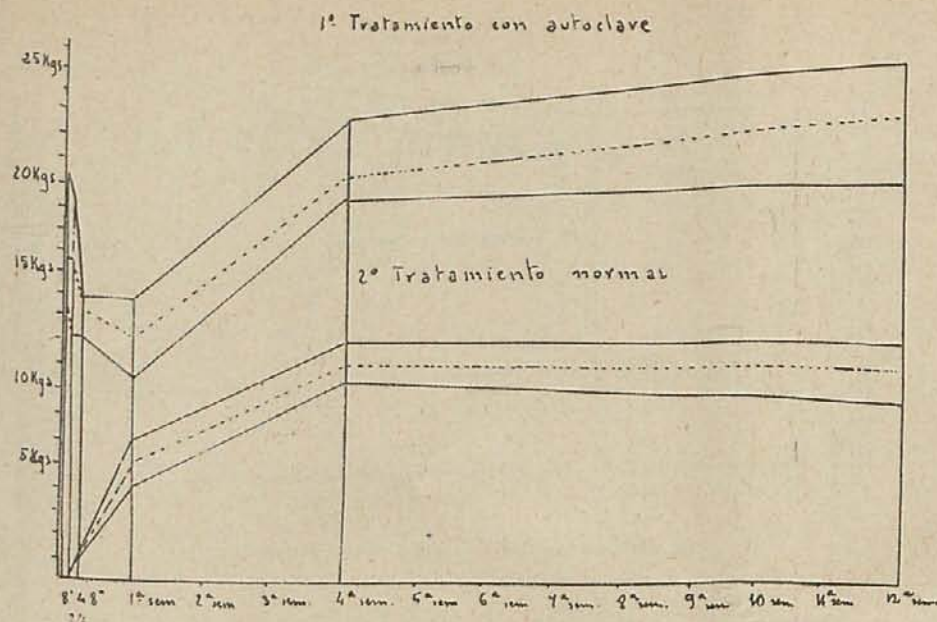
Fig. 3. Resistencia a la tracción de las probetas de cemento Portland
