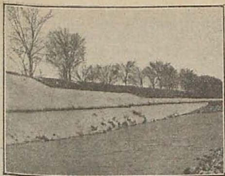
Adaptación de la colchoneta bajo la acción de las avenidas
