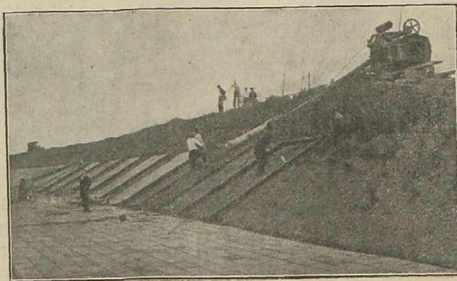
Construcción de las losetas de hormigón sobre la orilla
