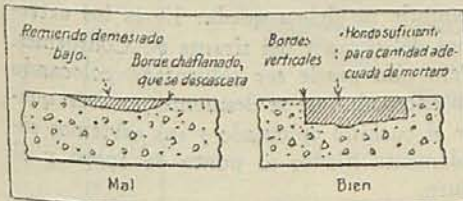
El método bueno y el malo de tapar un pequeño hoyo en un muro o piso de hormigón. A veces hay que usar un piso poco después de remendado. En tales casos tal vez la adición de cloruro de calcio al agua de la mezcla, ayude a dar prontamente resistencia al remiendo
