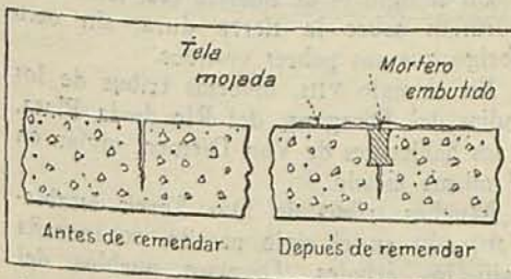
Reparación de una grieta como de 1 1/2 milímetros de ancho. En grietas muy finas, pueden limpiarse éstas con un chorro de agua y luego llenarse de lechada de cemento. Un método que ha dado buenos resultados en grietas finas horizontales, consiste en llenarlas de agua después de lavadas, y luego cerner cemento en el agua hasta que la grieta se llene.
