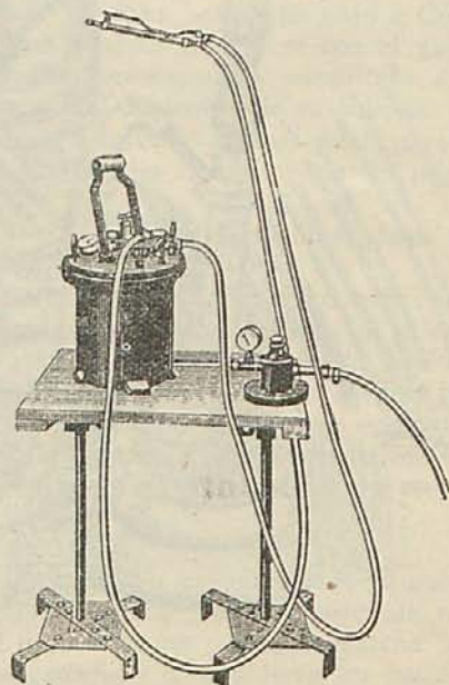
Fig. 3. — Aparato para pintar sistema «Brosse»
