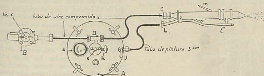
Fig. 4. — Esquemas del funcionamiento del aparato «Brosse»
