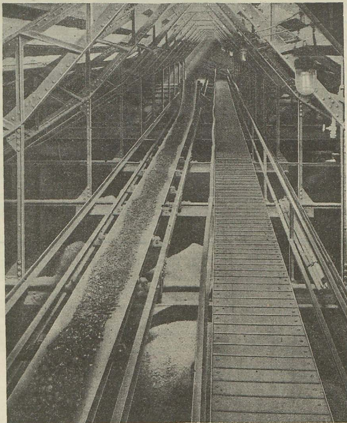
Vista de una correa "COBBETT" tres rayas negras, impregnada, de 559 7 / 8 mm. de ancho, que transporta carbón en la fábrica de La Catalana de Gas y Electricidad, de Barcelona
