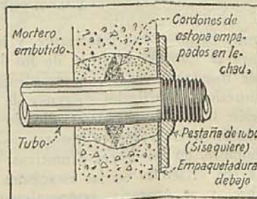
Instalación de un tubo a través de una pared vieja de hormigón. Si el tubo conduce vapor o agua caliente, debe encerrarse en un manguito, o disponer de alguna otra manera que le permita dilatarse y contraerse sin rajar el hormigón
