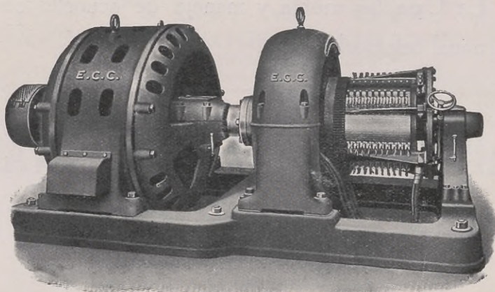
Motor generador de inducción D.C. para corriente monofásica de 125 kws. y 575 revoluciones por minuto.
