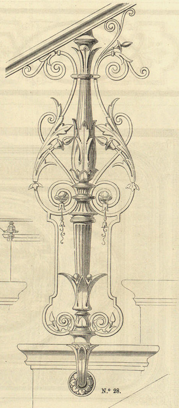
N.ºs 26 á 28. — Barandillas de hierro fundido. — F. de Hoven, arquitecto de Francfort.
