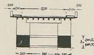
Fig. 7.—Puente de Ammer, en Echelsbach.
