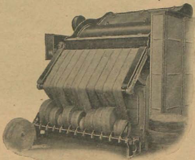
El gravat il·lustra l'extrem alimentari i part del costat d'engrenatge d'una carda fina semi-circular, alimentada per napes en lloc dels bots per a la cinta usual i doblant a 10 caps.
