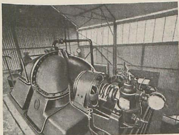
Grupo tubo-generator de 50 kilowatios de la fábrica de ensayo de Matanzas.
