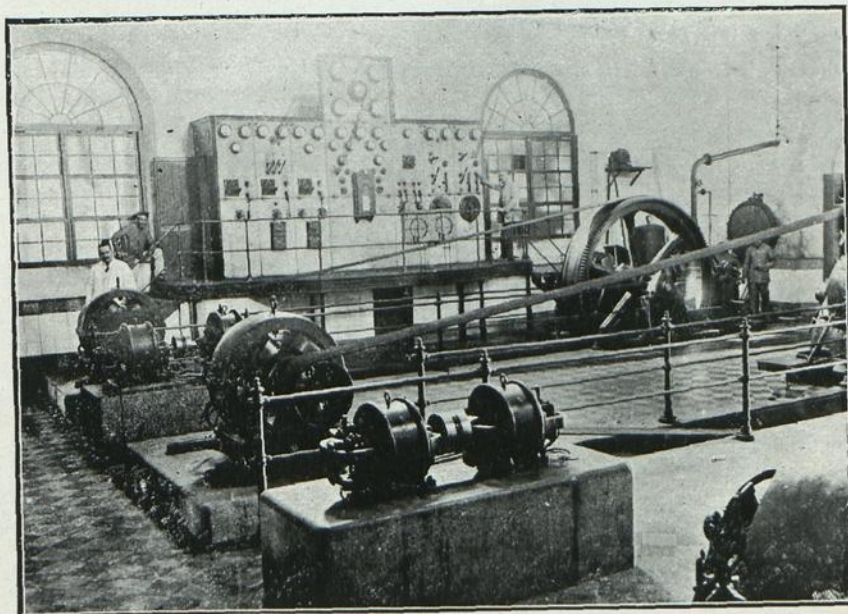
SALA DE MÁQUINAS Y CUADRO DE DISTRIBUCIÓN
