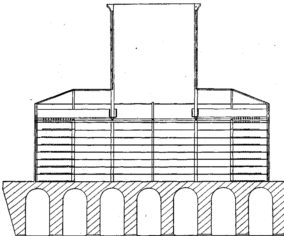
Figura 3. - Corte longitudinal.
