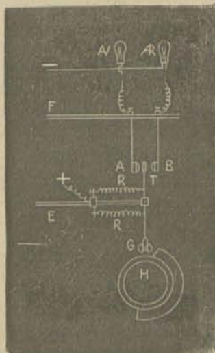
In Rador de vueltas eléctrico luminoso de Mr. Cadion, para medir la velocidad de rotación de las hélices de los barcos.
