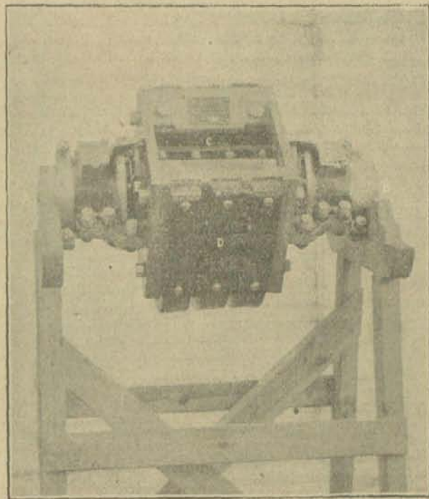
1.—Alternador acoplado al eje de la locomotora para la producción automática de la corriente.
