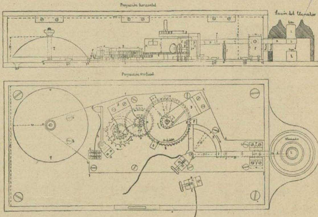
V.—Aparato de alarma de los coches.
