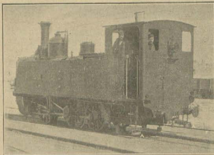
II.—Locomotora provista de los aparatos de electricidad.
