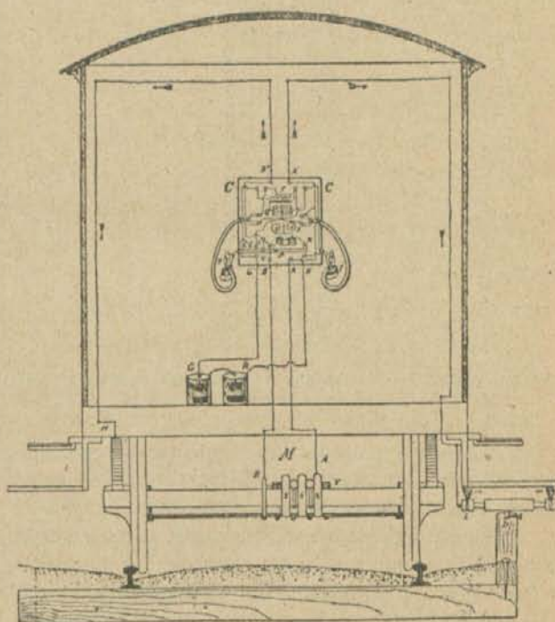
III.—Esquema del montaje de los aparatos en la máquina
