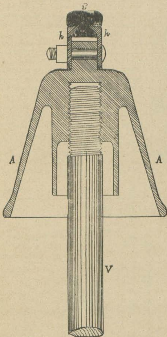
IV.—Sección del carril conductor de la corriente y de un aislador de celuloide.
