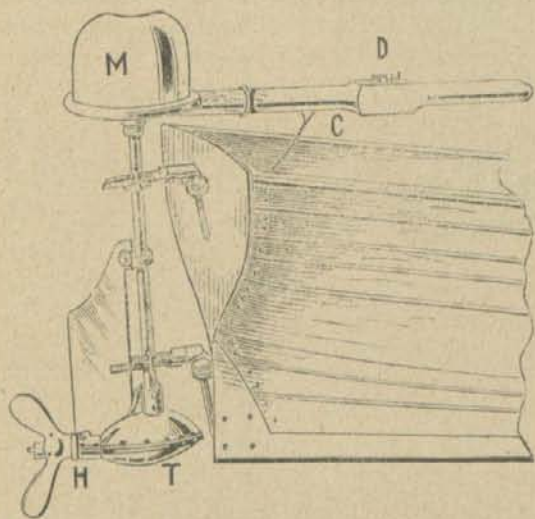
Propulsor de hélice eléctrica y portátil para embarcaciones de recreo.—M, pequeño motor eléctrico de un caballo; C, conductores eléctricos para dirigir la corriente de la batería de acumuladores colocados en la parte posterior; D, conmutador para ponerse en marcha; T, transmisión de movimiento; H, propulsor de hélice.
