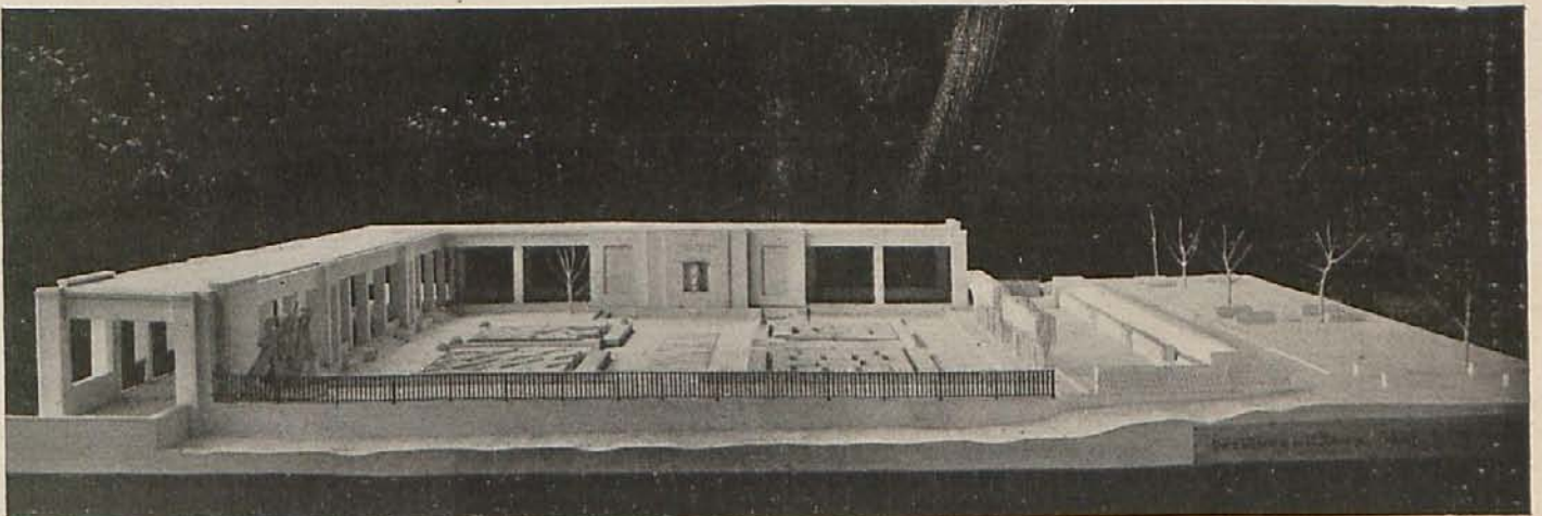
Vista en conjunto del proyecto para el monumento, que se emplazará en el Parque del Oeste, junto al Paseo de Camoens.
