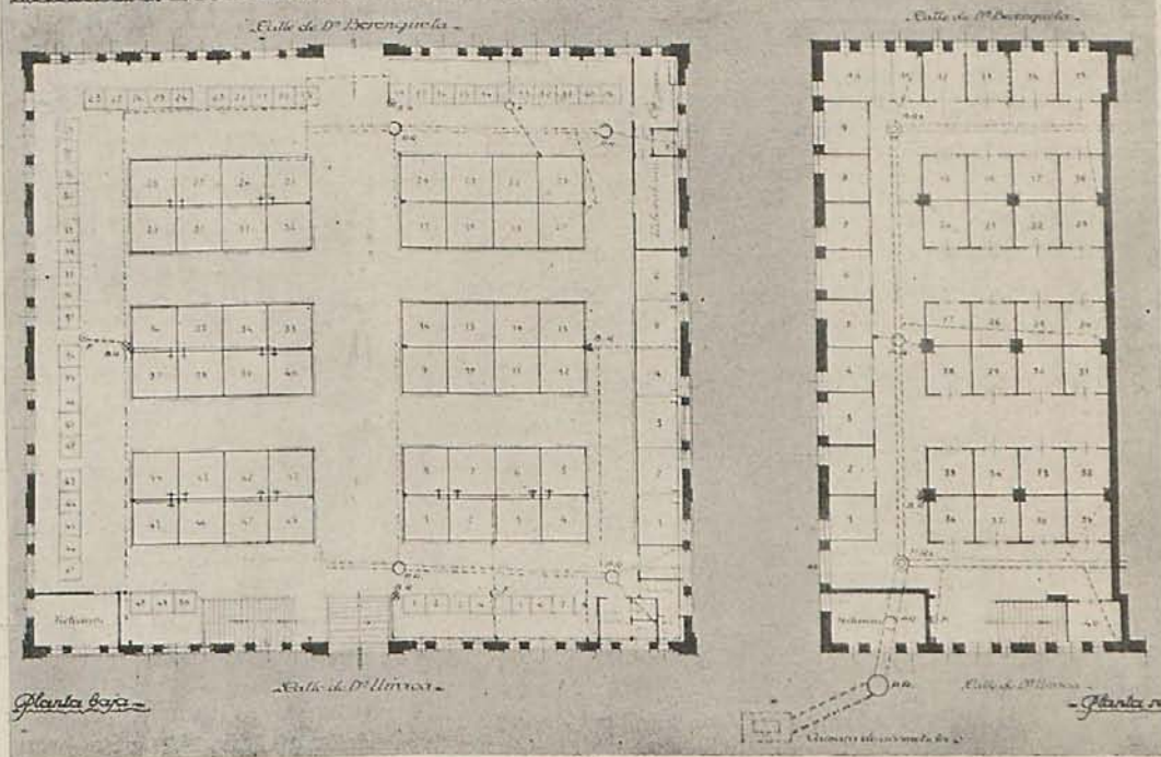
Plano de situación de los puestos locales y servicios de saneamiento del Mercado de Tirso de Molina. Escala 1:100.
