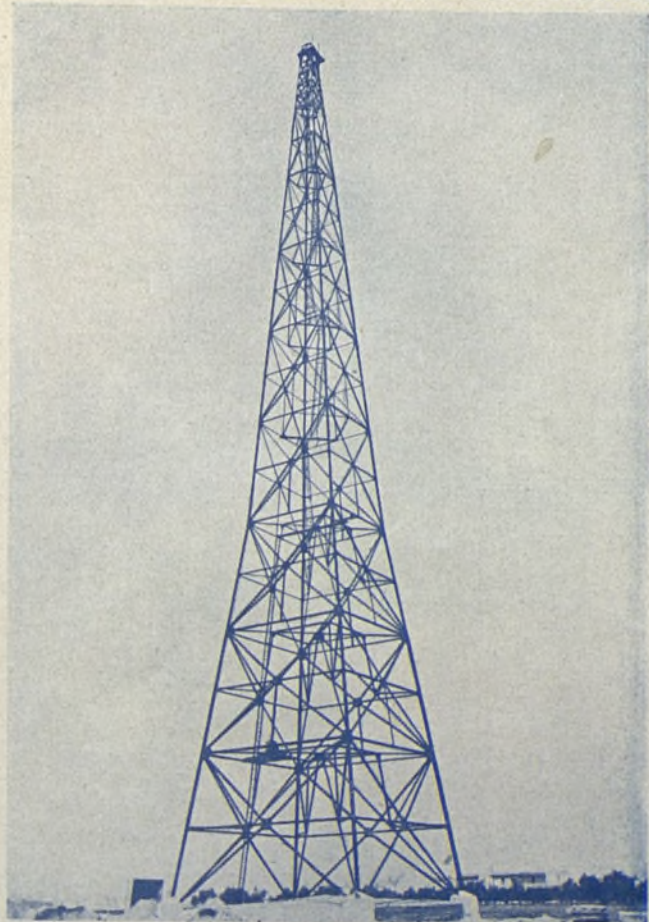
Torre metálica de 65 metros para RADIO ZARAGOZA
