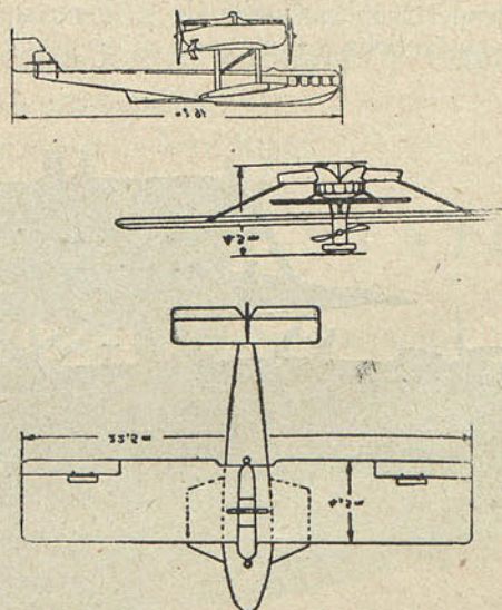
Croquis esquemático del hidroavión Dornier "Wal" ("Plus Ultra").
