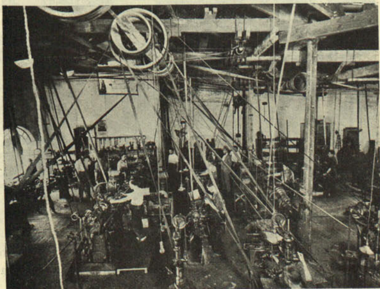
Secciones de torneado y ajuste
