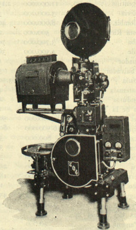
El gran aparato «Super Model», construido a base de circuitos dobles, que da la seguridad al empresario de la imposibilidad de sufrir paro alguno por avería
