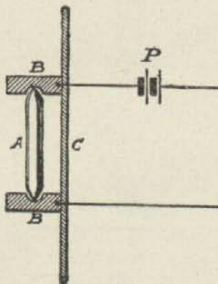
Figura 5. a Micrófono Hughes.
