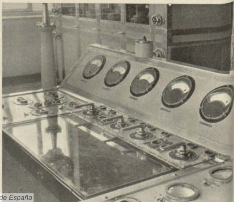
Pupitre de control de una moderna estación Marconi de radiodifusión
