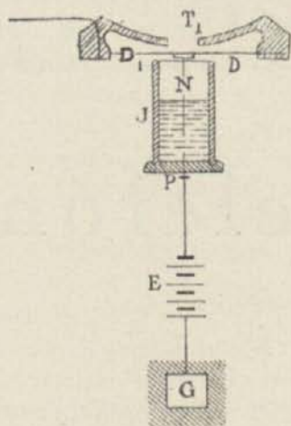
Figura 1. a Micrófono Elisha Gray.
