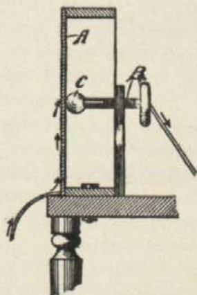
Figura 3. a Micrófono Berliner.
