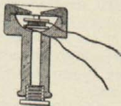
Figura 4. a Micrófono Edison.
