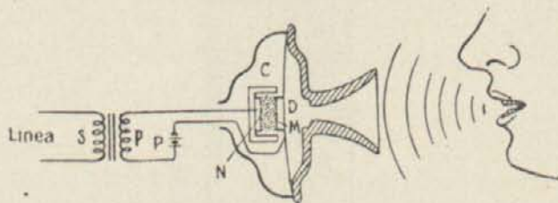
Figura 8. a Micrófono de granalla de carbón.
