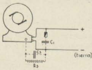
Figura 7. a Primera variante
