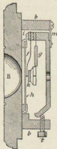
Figura 6. a Micrófono Black.
