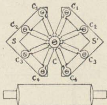
Figura 7. a Micrófono Grower.
