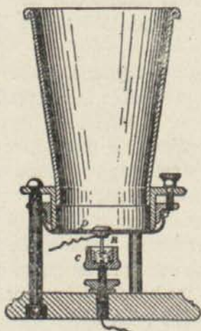
Figura 2. a Micrófono Bell.
