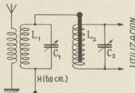
Figura 3.ª Circuito preselector con el dispositivo de acoplo expuesto en estas líneas.
