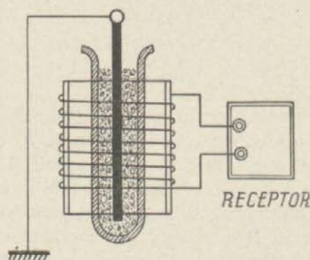
Figura 1.ª Idea esquemática del dispositivo experimental para establecer acoplamientos por difusión.
