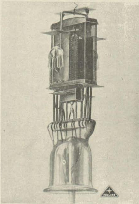
La lámpara «binodo» E444.
