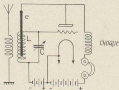
Figura 2.ª Circuitos de placa y rejilla de una lámpara detectora acoplados por difusión.
