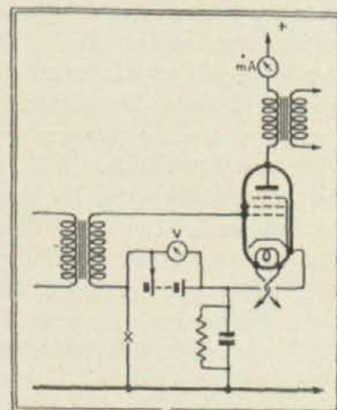
Dispositivo para medir la polarización automática introducida por una resistencia, sustituyéndola por una batería de pilas.
