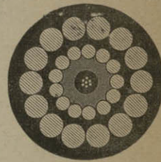
Cable submarino.
