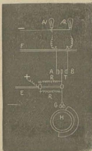
In Rector de vueltas eléctrico luminoso de Mr. Cadion, para medir la velocidad de rotación de las hélices de los barcos.
