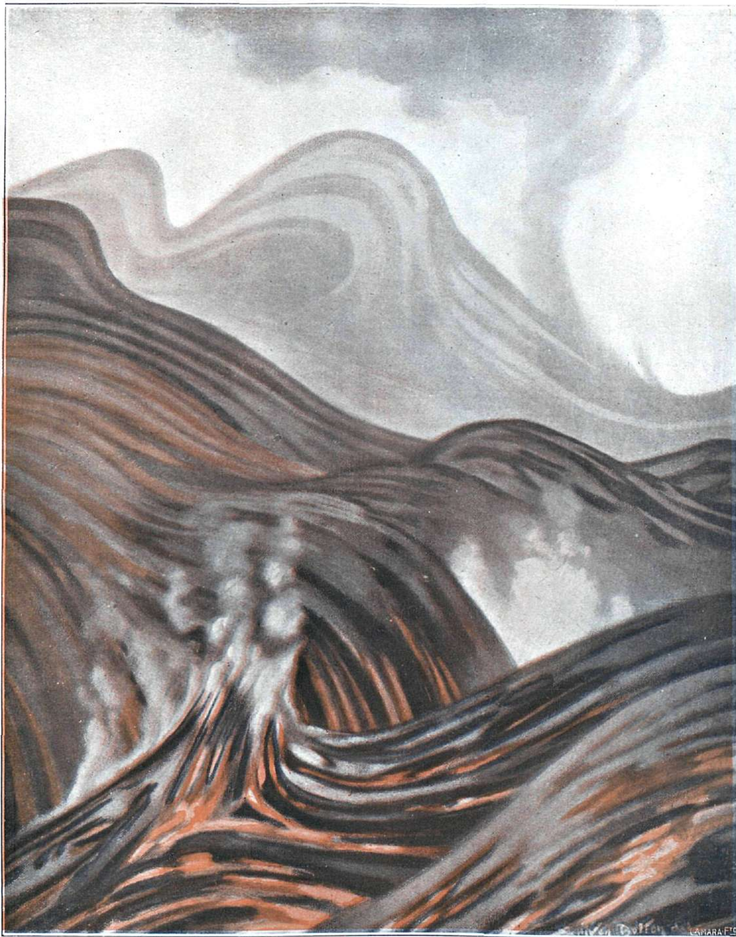
Aspecto que debe presentar la superficie del planeta Júpiter, según las más recientes observaciones
