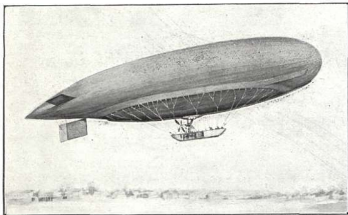
Dirigible alemán P-III , flexible, de 10,000 m. 3 ; longitud, 84 m.; diámetro, 15'5 m.; motores, 400 H. P.; velocidad, 65 kilóm. Construido en 1911
