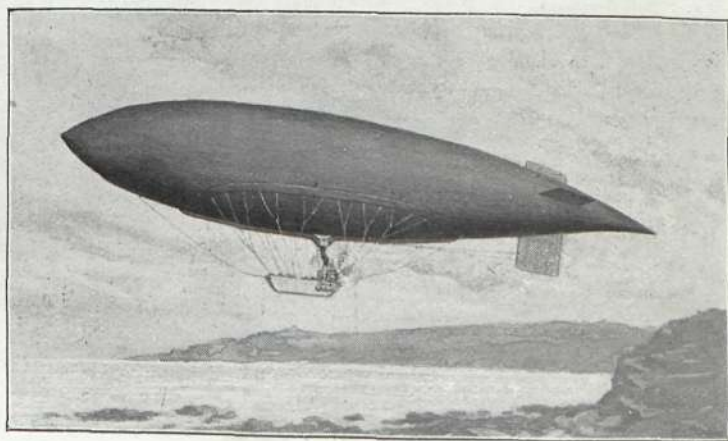
Dirigible inglés Parseval , flexible, de 8,800 m. 3 ; longitud, 84 m.; diámetro, 15 m.; motores, 360 H. P.; velocidad, 68 kilóm. Construido en 1913
