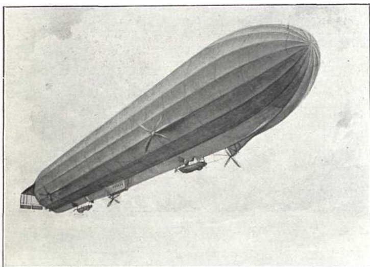
Dirigible alemán Z. VI , rígido, de 19,500 m. 3 ; longitud, 141 m.; diámetro, 14'8 m.; motores, 540 H. P.; velocidad, 77 kilóm. Construido en 1913
