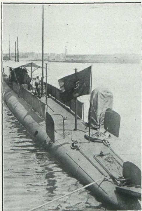
El sumergible portugués «Espadarte» Primer buque de esta clase que ha visitado nuestro puerto.—(Fotog. Carlos Perez)
