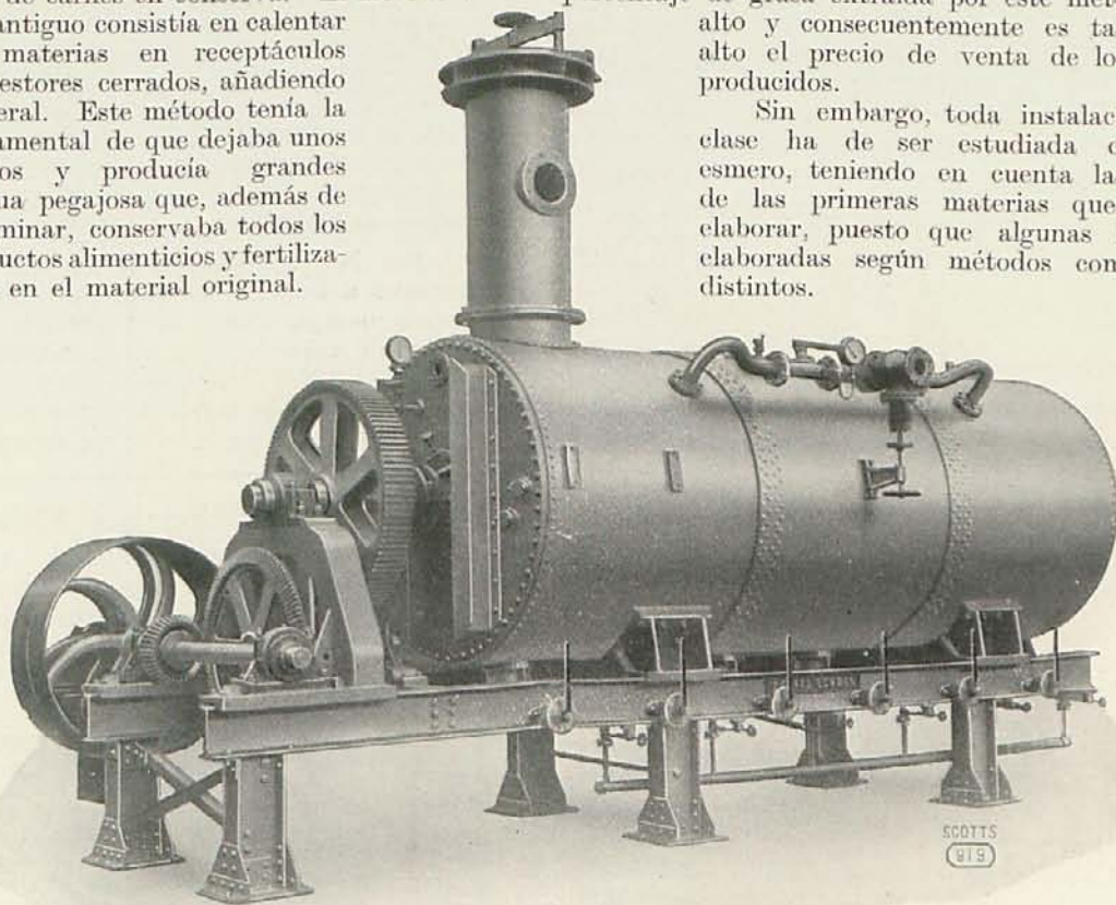
Máquina "Scott" para la extracción de grasas.
