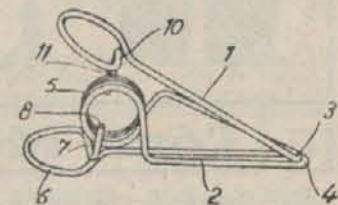
Pinza con muelle de una sola pieza.
