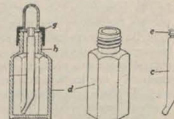
Frasco con pipeta que se llena por aspiración de una cápsula de goma.
