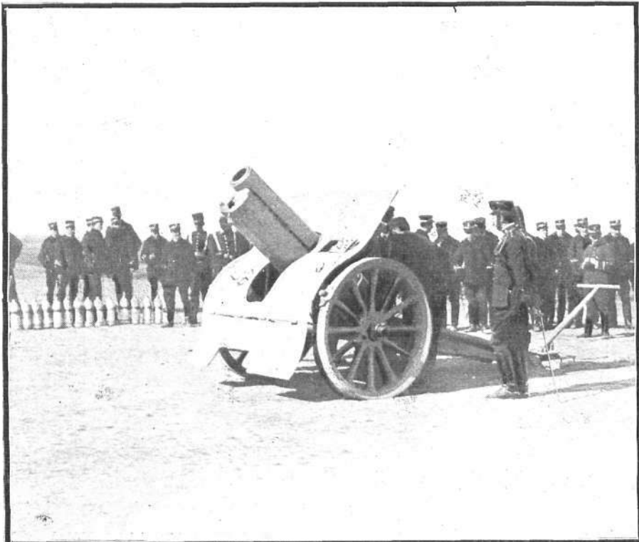
SEGOVIA. PRUEBAS DEL NUEVO OBÚS DE 15 CENTÍMETROS Y TIRO RÁPIDO, SISTEMA SCHNEIDER Fot. Duque
