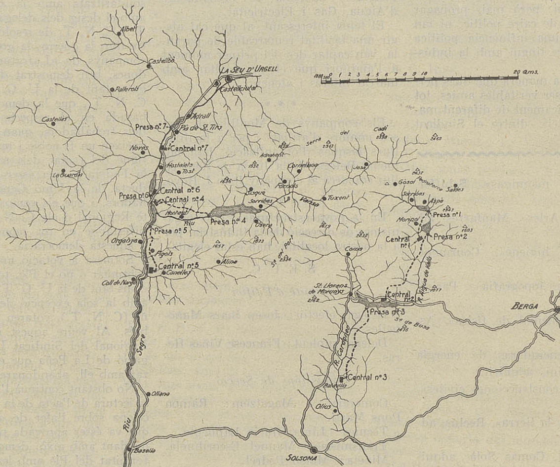
Pla de la conca total de cap ació dels aprofitaments hidro-elèctrics dels rius La Vansa, Aigua de Valls, Cardoner i parcial dels del Segre amb l'emplaçament de les preses, embassaments, canals de conducció i centrals
